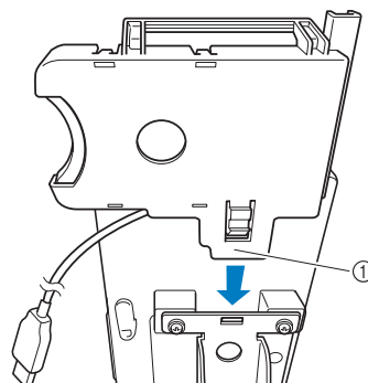
① Brazo
