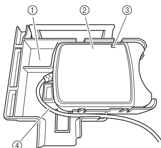
① Soporte del lector de tarjetas ② Lector de tarjetas de bordado ③ Indicador ④ Cable del lector de tarjetas
