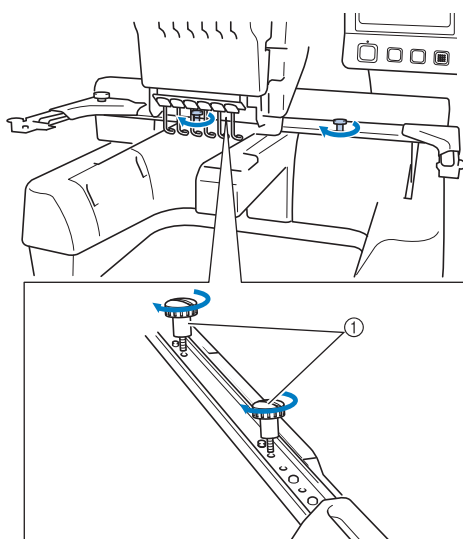
① Tornillos de mariposa
