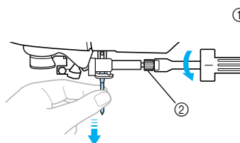
① Destornillador
